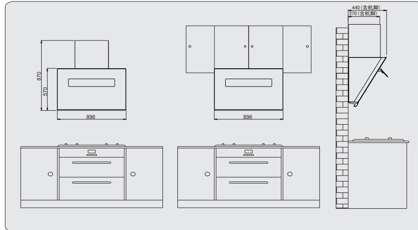
CXW-230-PH1G926C-SDBT 安装示意图:
