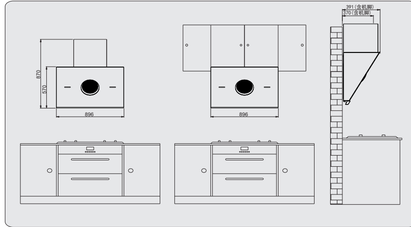
CXW-230-PH1G919C-SDBT 安装示意图:
